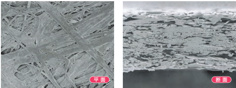
タイベック®を構成する強靱な極細ポリエチレン繊維(約300倍)
