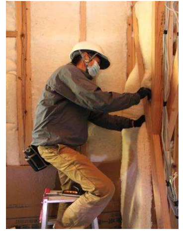
③ 両サイドをタッカーで固定します。
